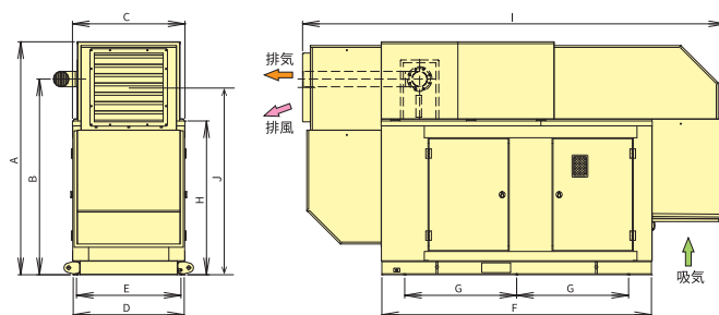
DCA-225SPGF(三菱エンジン機)
