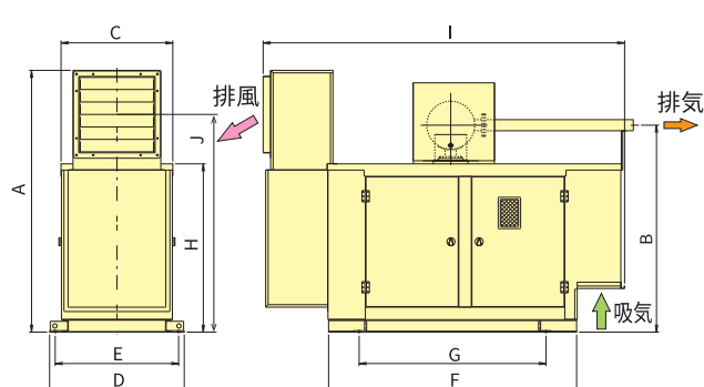
DCA-65SPGF(三菱エンジン)
