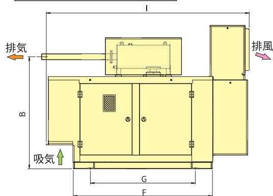
DCA-65SPGF(いすゞエンジン)
