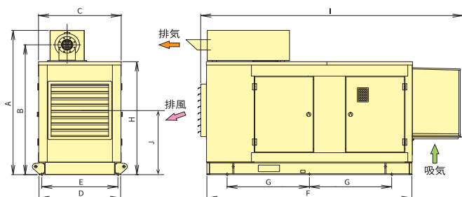
DCA-225PGF(コマツエンジン機)・255PGF
