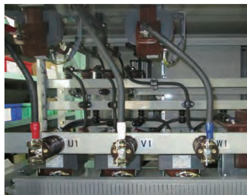
D (高圧中継端子台)
