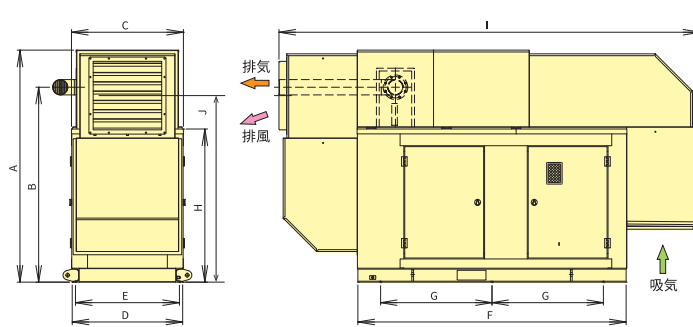
DCA-225SSGF(三菱エンジン機)
