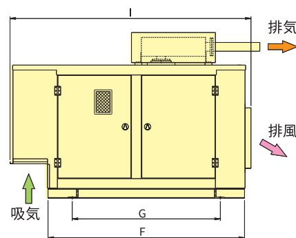
DCA-65PGF(いすゞエンジン機)
