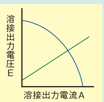
アーク長が長くなり電圧が上昇することで、電流が減少
