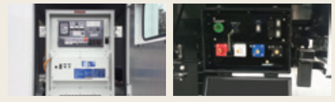
操作盤・出力端子(DCA-60SGC-I)
