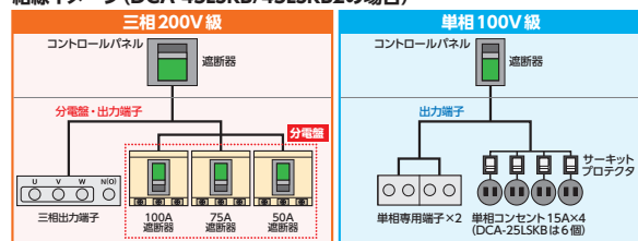
結線イメージ (DCA-45LSKB/45LSKB2の場合)
